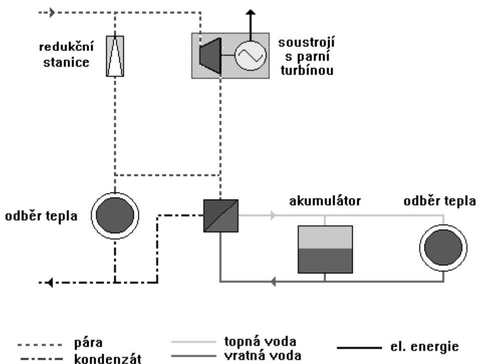
Obrázek 3 Parní kogenerace
