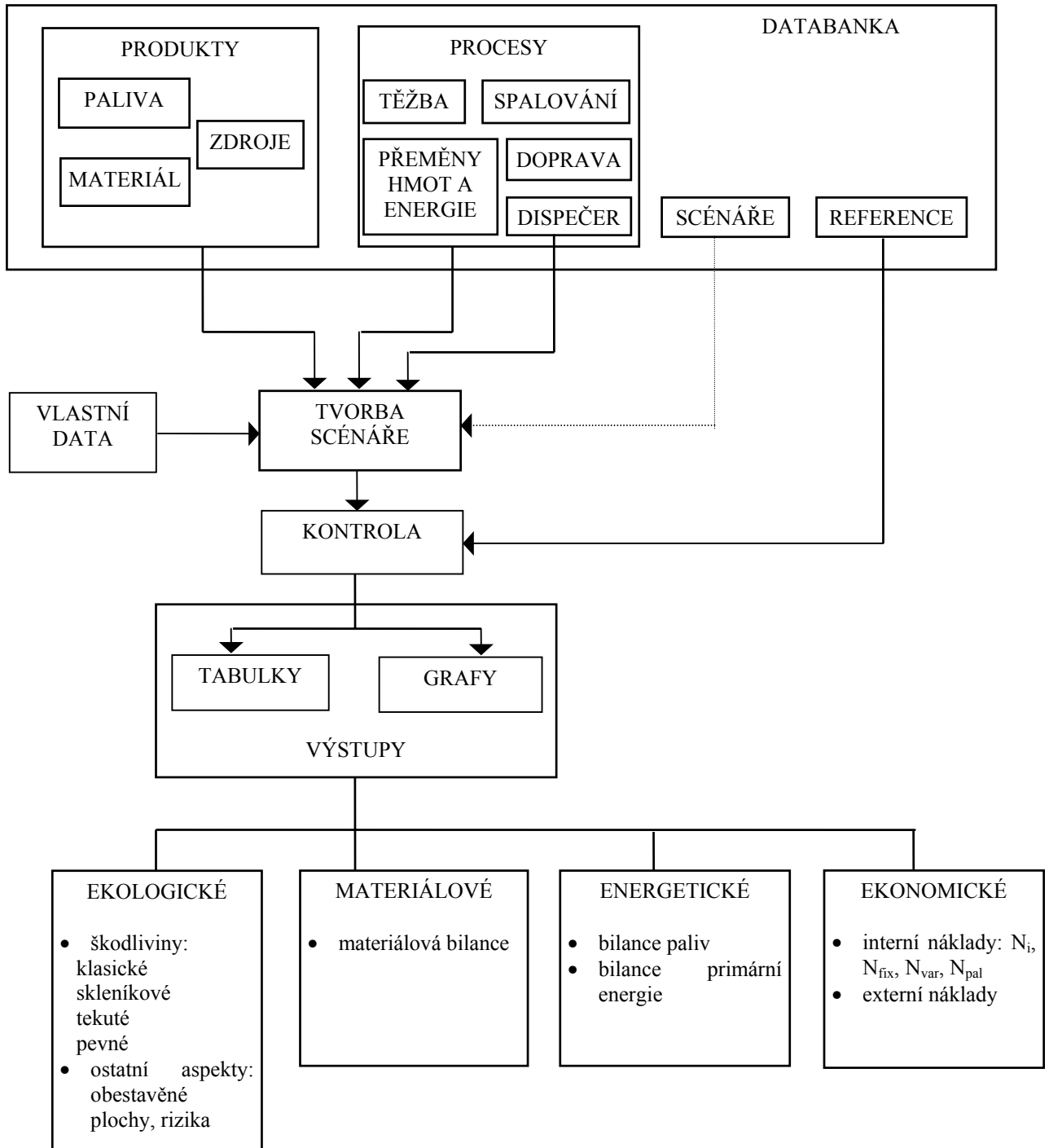
Obr.1 Funkční schéma GEMIS
